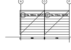
KLADACSKÝ PLÁN C-KAZETY POHLAD VÝCHODNÝ STĚNA „23“
