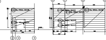
KLADACSKÝ PLÁN C-KAZETY POHLAD VÝCHODNÝ STĚNA „1“ STĚNA „N“ STĚNA „22“
